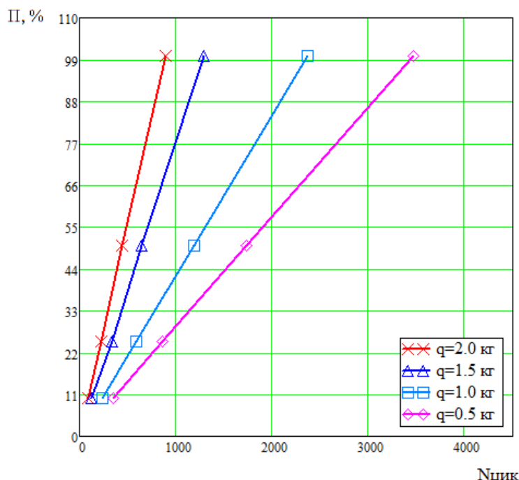
Рисунок 2 - Зависимости потери прочности рыболовной нитки ПА 187 текс×12 ( \Pi , %) (сухой) от количества циклов истирания ( N_{\text{цикл}} ), при различной загрузке сбегающих ветвей ( q ), шероховатость истирающей поверхности W = P100 , \Pi = f(N_{\text{цикл}})
