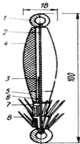
Рисунок 3.3 – Кальмароловный крючок джигер типа зорори, применяющийся в вертикальных пелагических ярусах:
