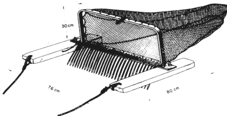
Рисунок 6.3 - Ползчатая драга
