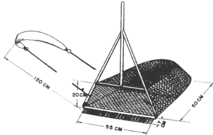
Рисунок 4.5 - Ручная драга
