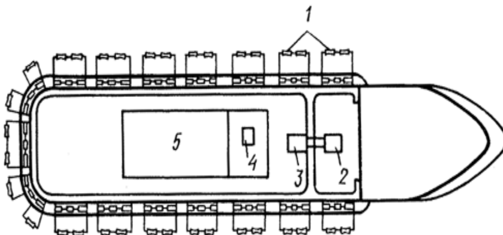
Рисунок 3.7 - Схема компоновки главной палубы специализированного 99-тонного судна для лова кальмаров вертикальными снастями со сдвинутым нос ходовым мостиком: 1 - кальмароловные лебедки; 2 - накопитель сырья; 3 - сортировочное отделение; 4 - подготовительное отделение; 5 - морозильное отделение
