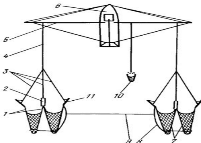
Рисунок 2.3 - Схема буксировки четырех тралов для лова креветок:
