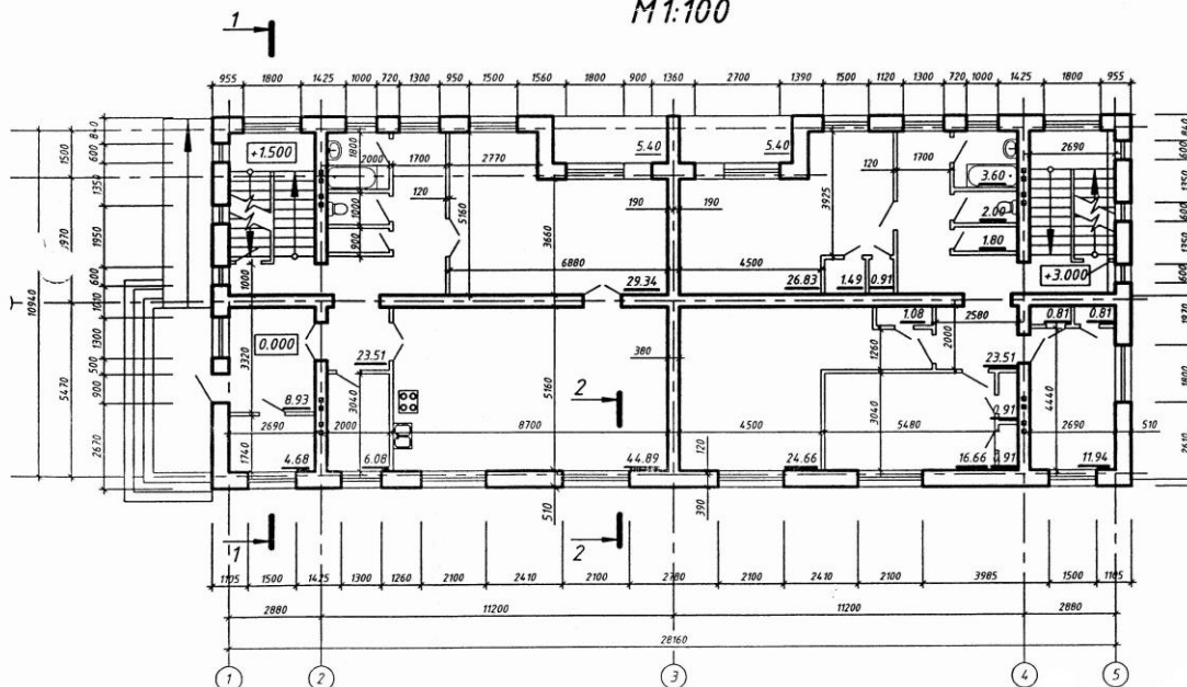
План на отм. 0.000 в осях 1-3 и на отм. +3.000 в осях 3-5 М1:100
