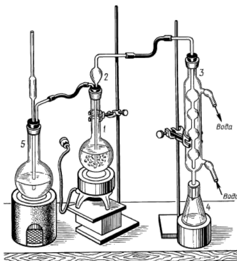
Рисунок 3.1 – Прибор для отгонки летучих кислот
