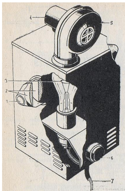
Рисунок 6.2 – Овоскоп И-11 А:
