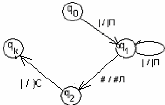
Рис. 0.2. Граф алгоритма
