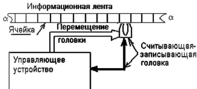
Рис.1. Машина Тьюринга
